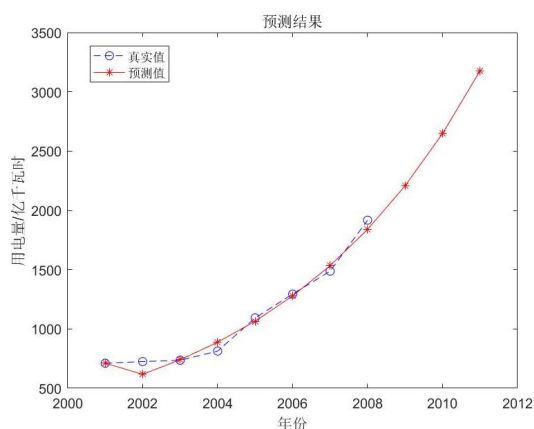
图 1 传统 GM(1,1)模型数据拟合结果
