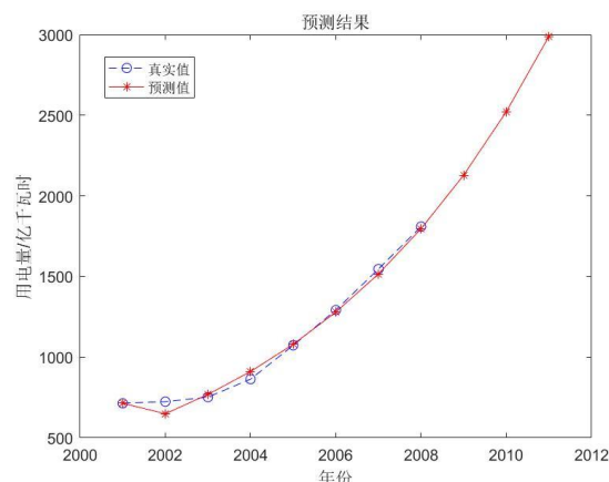
图 2 改进 GM(1,1)模型数据拟合结果
