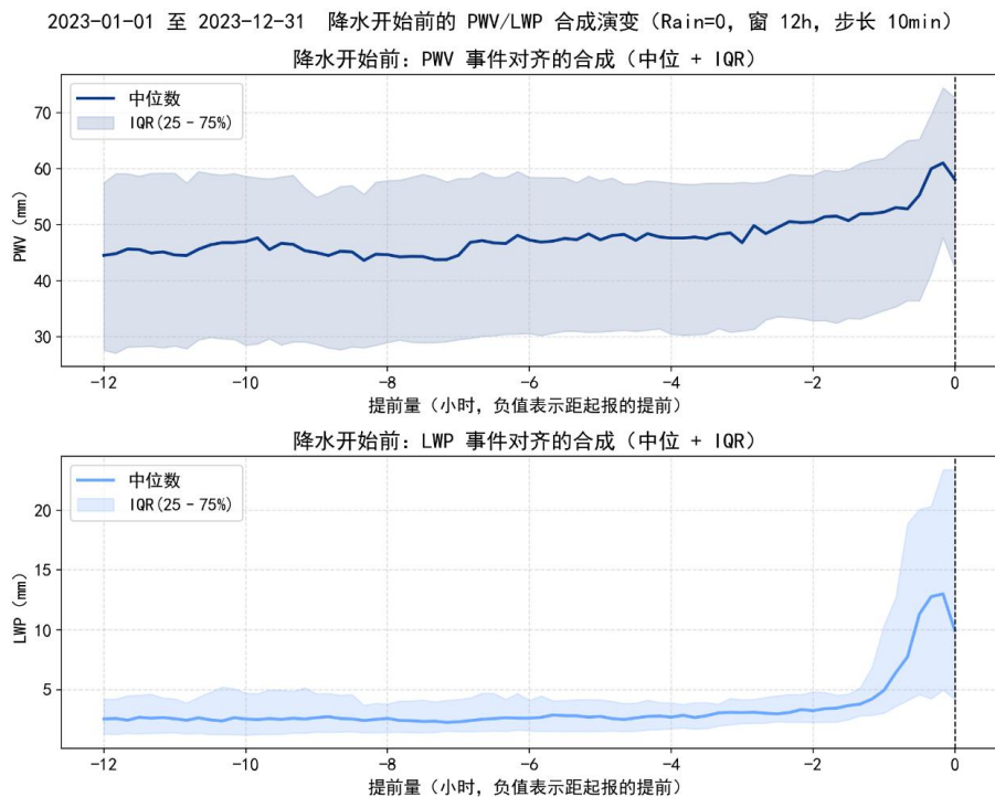
图 1: 降水事件前 12 小时整层可降水量 (PWV) 与云液态水路径 (LWP) 的合成演变
