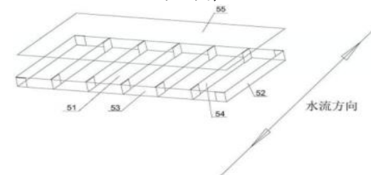
图 3 生态河道的防渗结构中位于边坡的雷诺护垫的摆放示意图；
