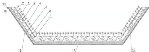
图 1 是生态河道的防渗结构的横断面图；
